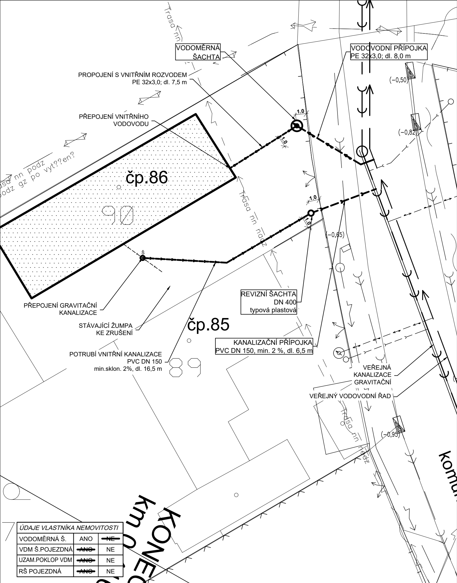
Rodinný dům č.p.86 SITUACE 1:200
