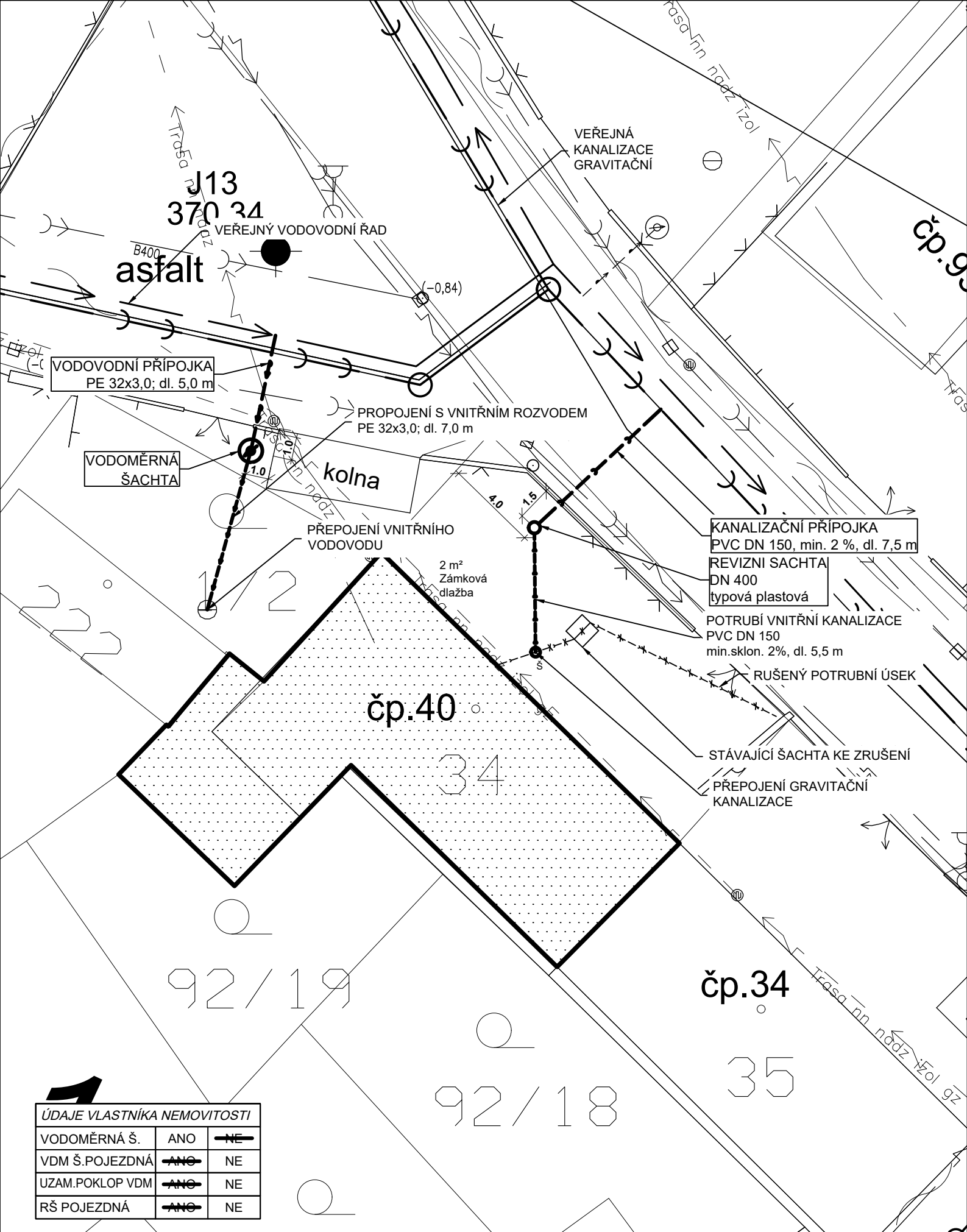
Rodinný dům č.p.40 SITUACE 1:200
