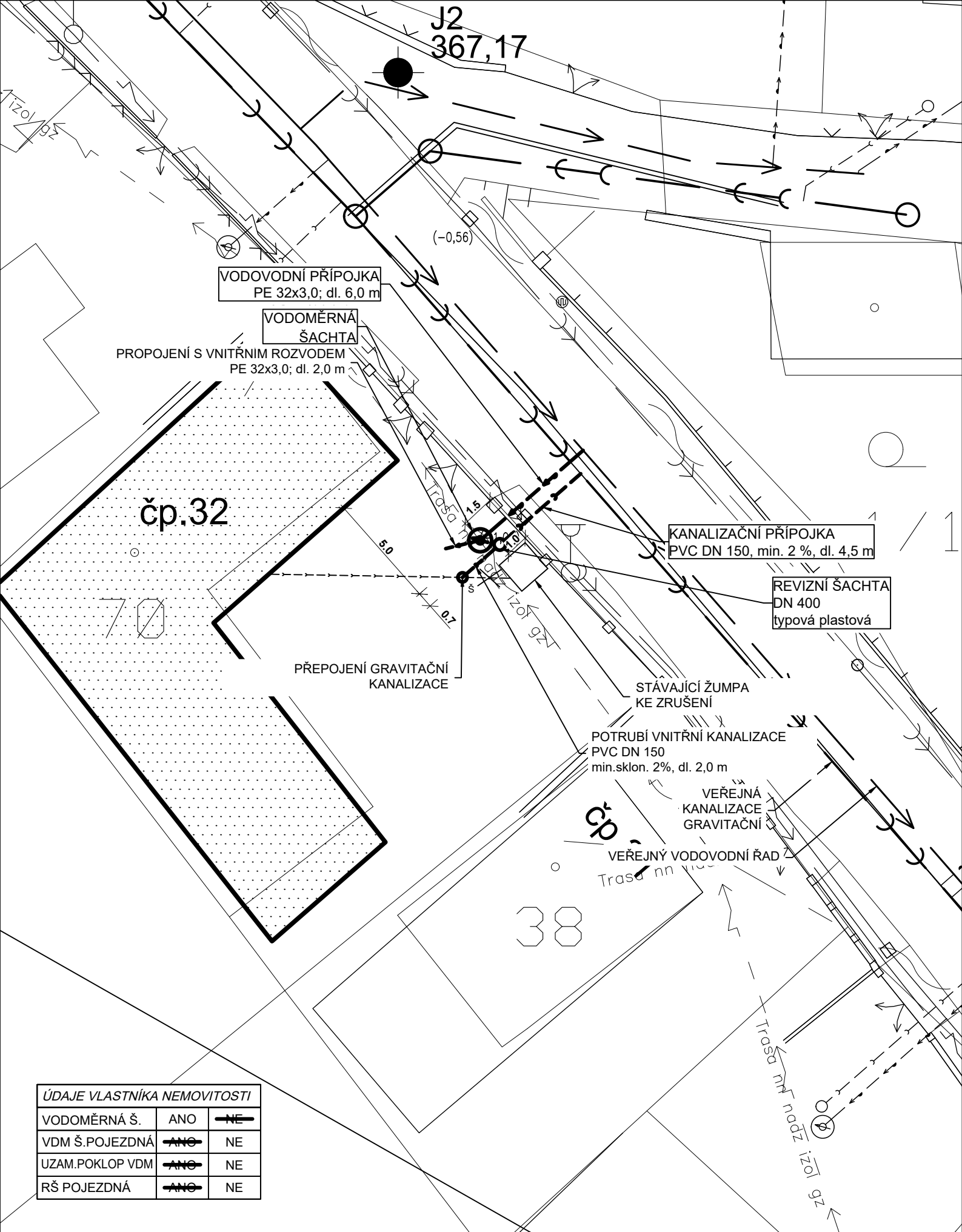
Rodinný dům č.p.32 SITUACE 1:200
